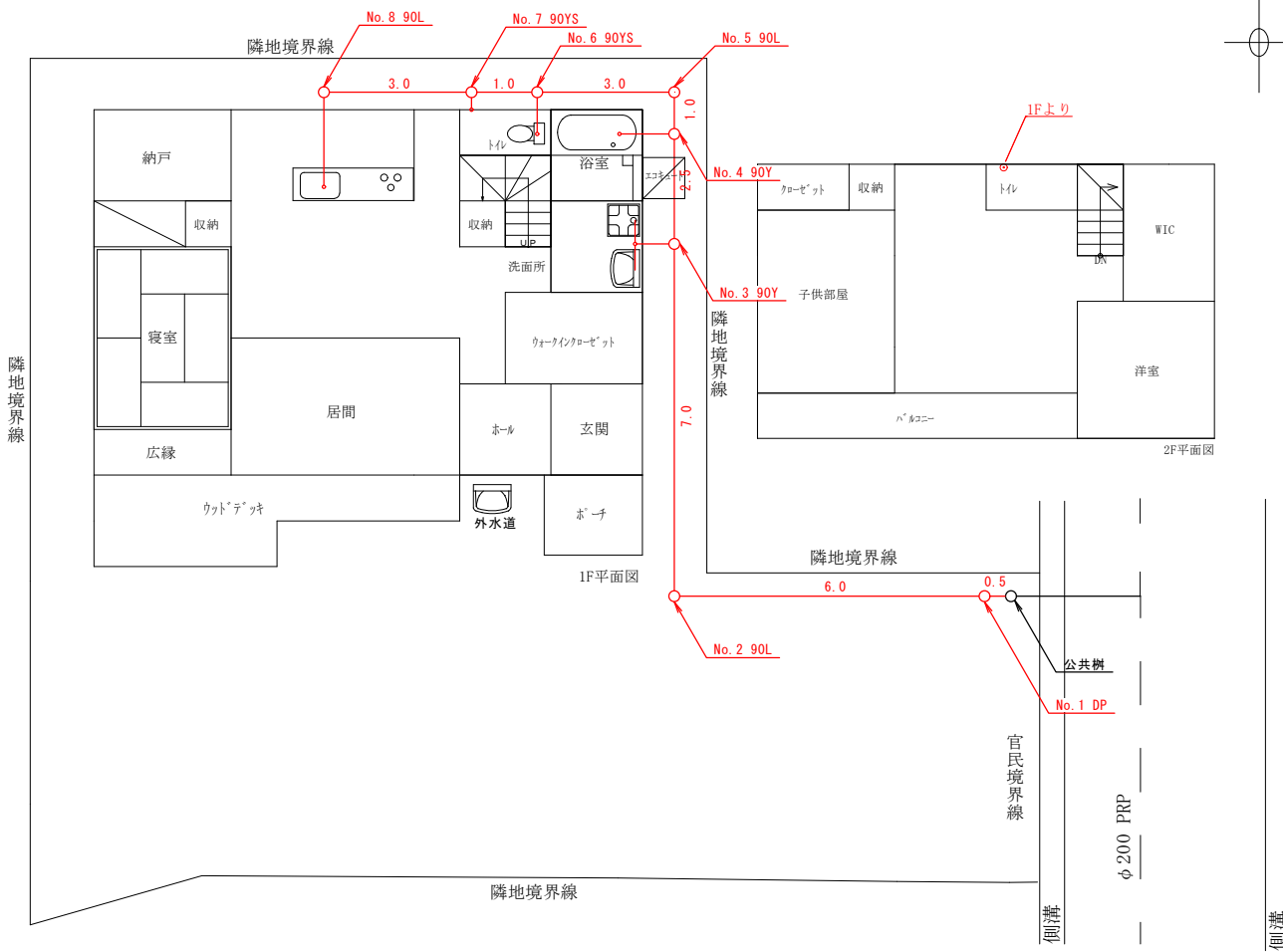
平面縦断図
